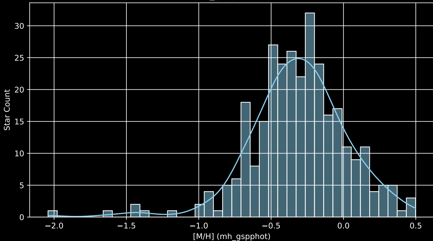
GALAH DR4 Field: [354] [M/H] (mh_gspphot) (n= 302)
