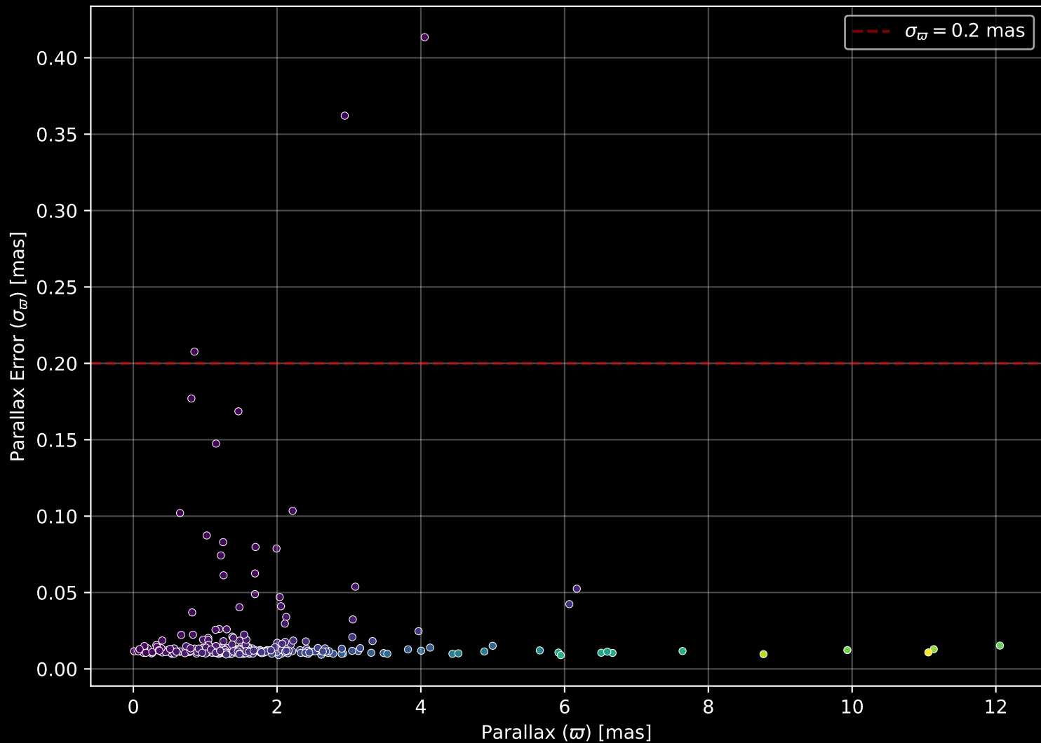
GALAH DR4 Field: [354] Parallax Quality (n= 303)
