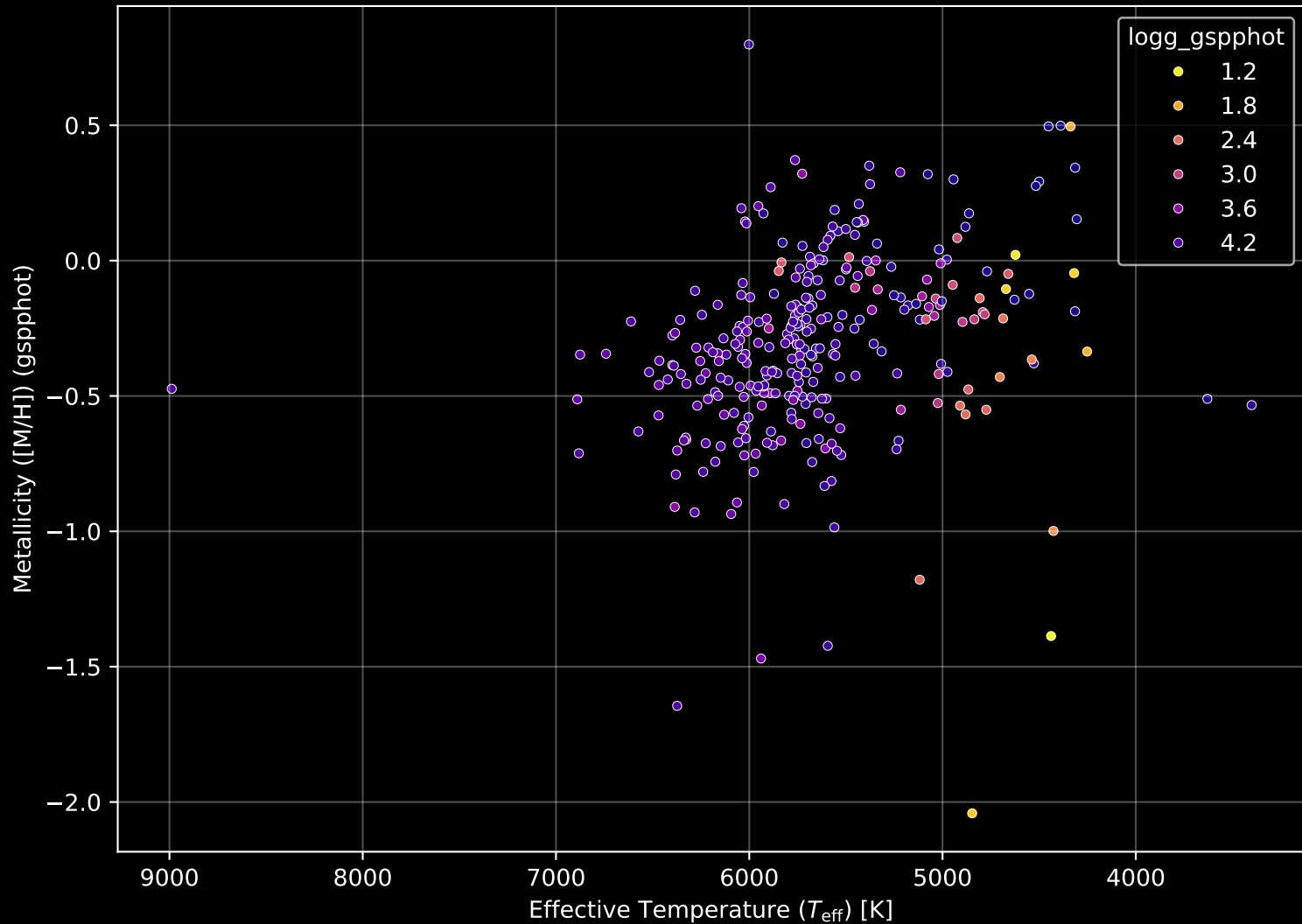
GALAH DR4 Field: [354] Stellar Population Parameters (n= 303)
